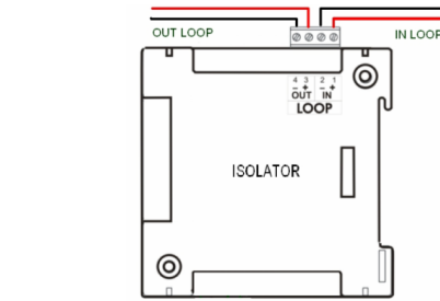
Modulo Aislador: Entrada Loop borne 1 y 2 Salida Loop borne 3 y 4
